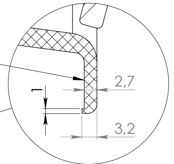
SZCZEGÓŁ C SKALA 2 : 1
